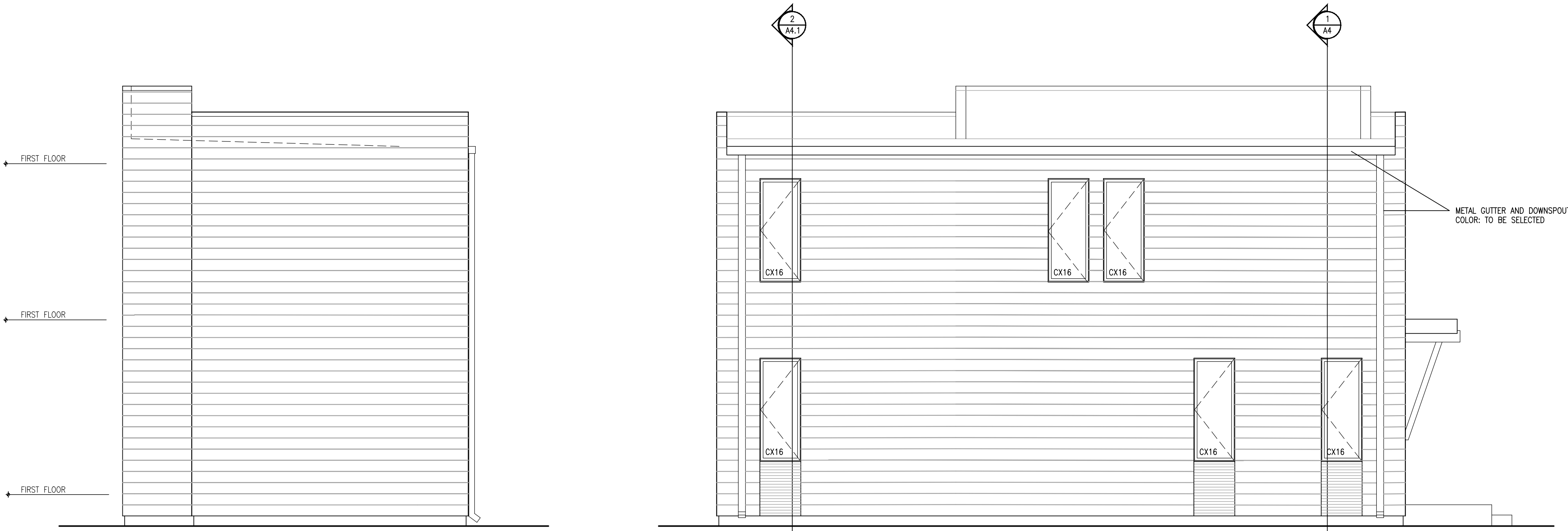
④ BACK ELEVATION SCALE: 1/4"=1'-0"
